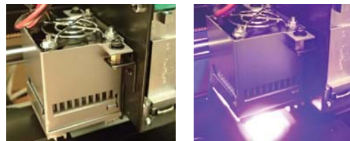
小型 UV インクジェットプリンター組込み例
